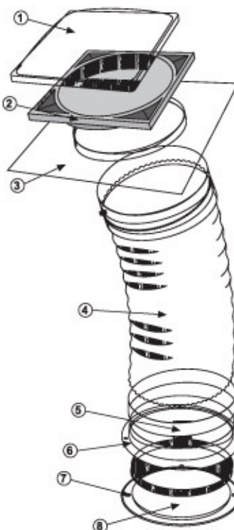
Kit de ventilación
