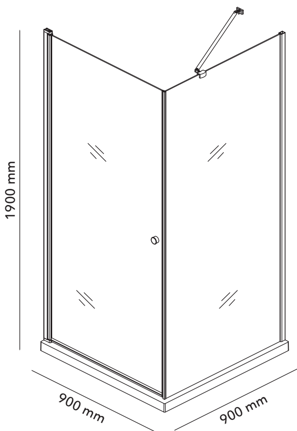
INSTALACIÓN IZQUIERDA
