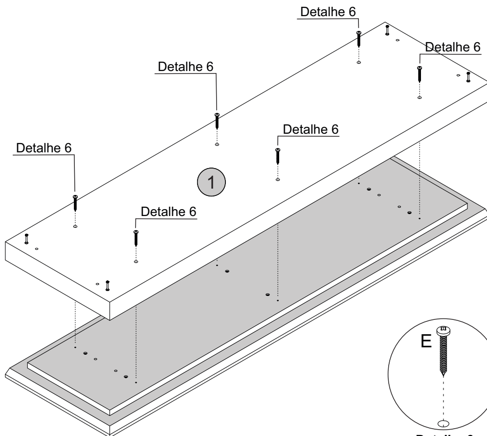
Detalhe 6 Detail/Detalle
