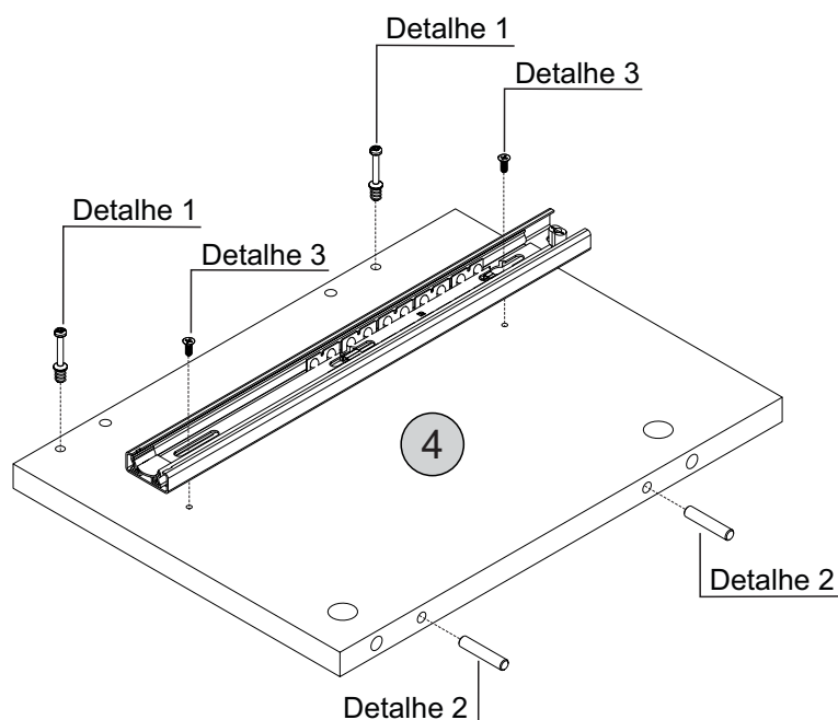
Detalhe 2 Detail/Detalle
