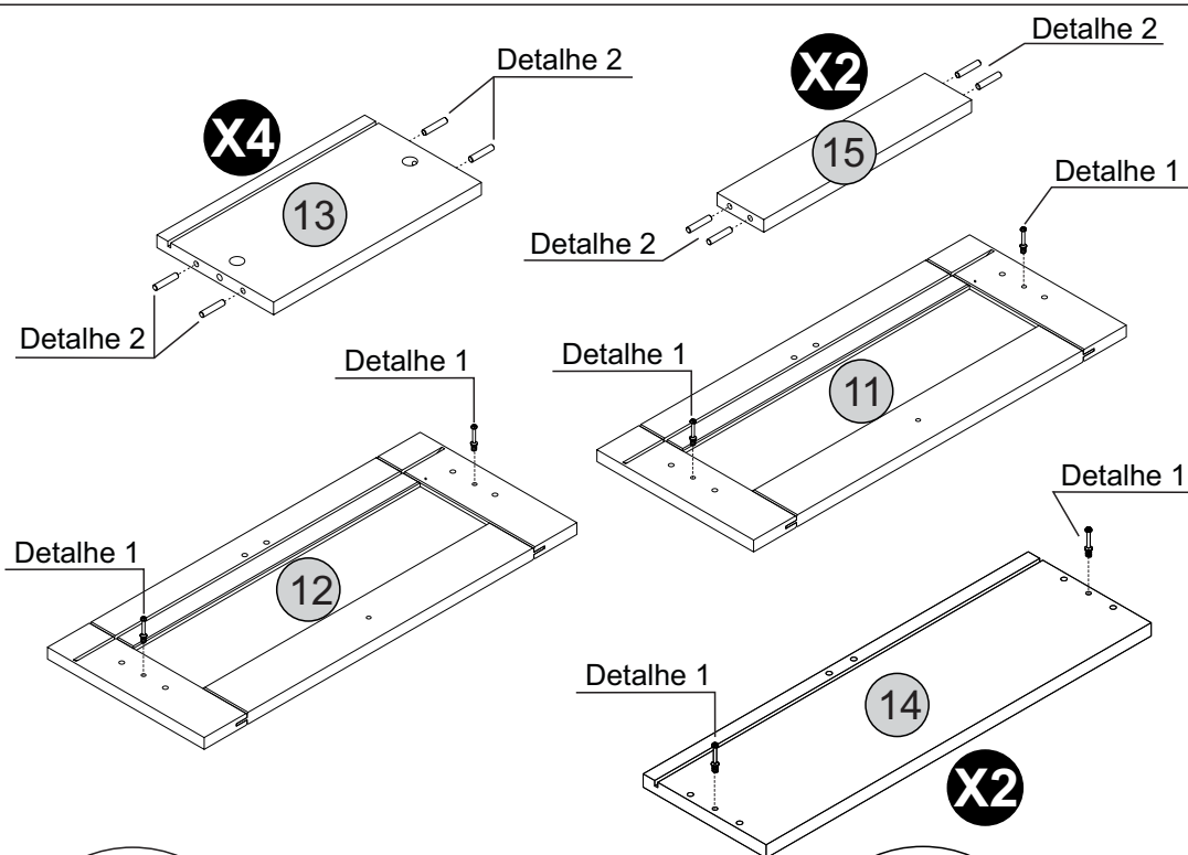
Detalhe 2 Detail/Detalle
